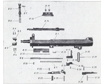
MG 34, Einzelteile: Gehäuse
